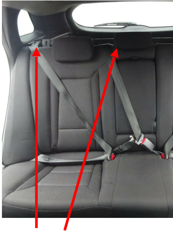
El retractor está unido al chasis del vehículo dentro de la estructura del asiento al final del cinturón de hombro.
